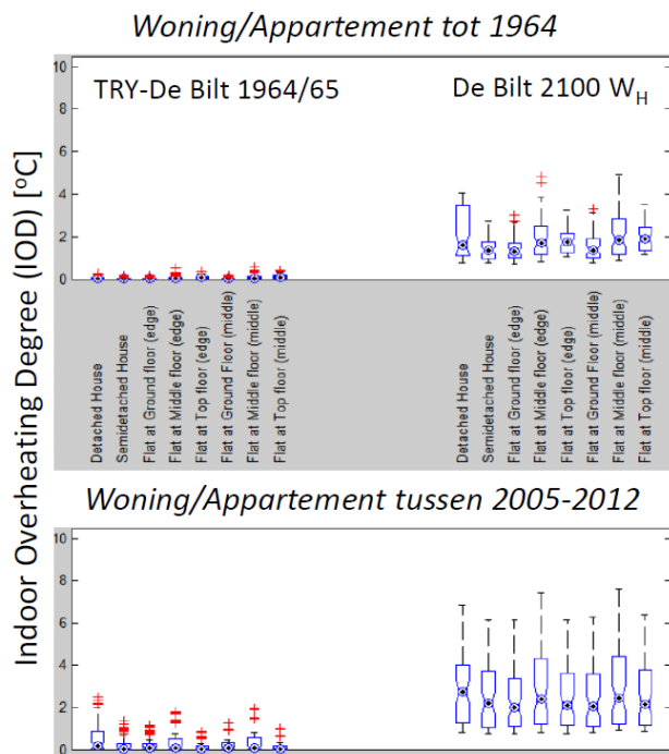
Figuur 1. Risico op oververhitting voor verschillende typen woningen van voor 1964 en meer recent tussen 2005-2012, uitgaande van typische uitgangswaardes voor de bouwstijl. IOD = Indoor Overheating Risk; combineert intensiteit/amplitude en frequentie van de oververhitting inclusief het gebruik van de ruimtes over de dag. [7]
