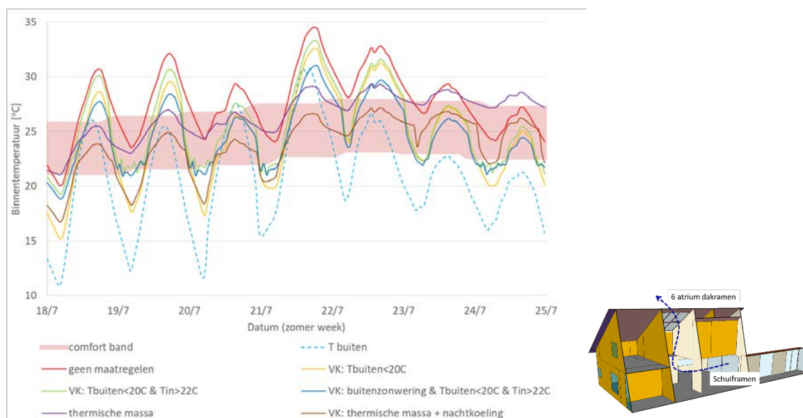
Figuur 2. Voorbeeld van het gesimuleerde temperatuurverloop in een woning tijdens een warme zomerweek en het gebruik van verschillende maatregelen om de temperatuur binnen te verlagen (VK: Vrije Koeling). [8]
