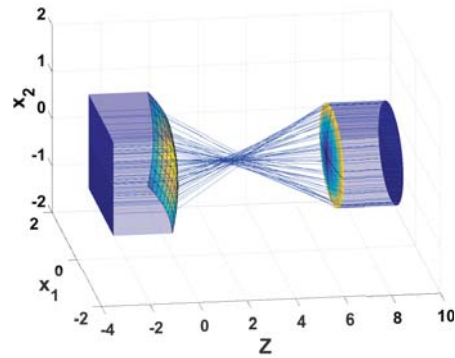
(d) Two lenses, c-concave case.
