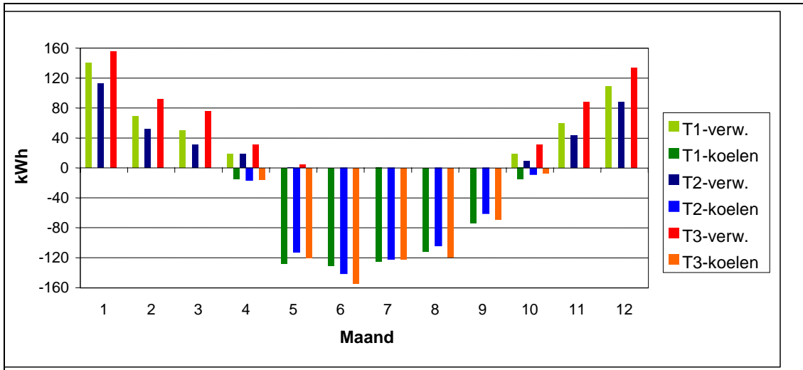
Figuur 7. Maandelijke energiebehoefte voor verwarmen en koelen van het kantoor bij west oriëntatie in Nederland.
