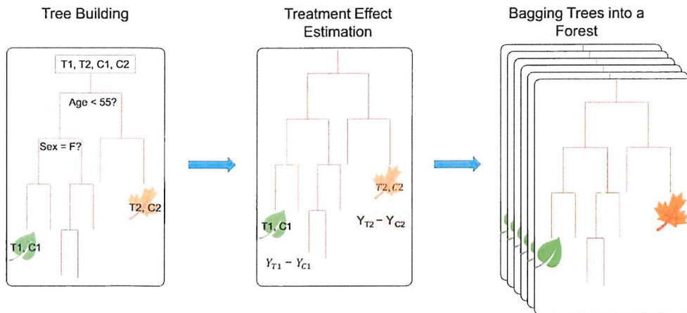
FIGUUR 3 ► CAUSAL FOREST
