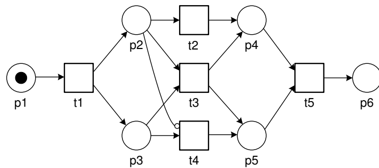
(d) Extended Petri net with inhibitor arcs
