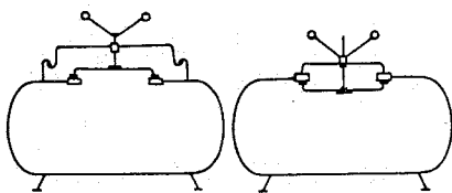
Figuur 6 Zelfafsluitend mangatdeksel
