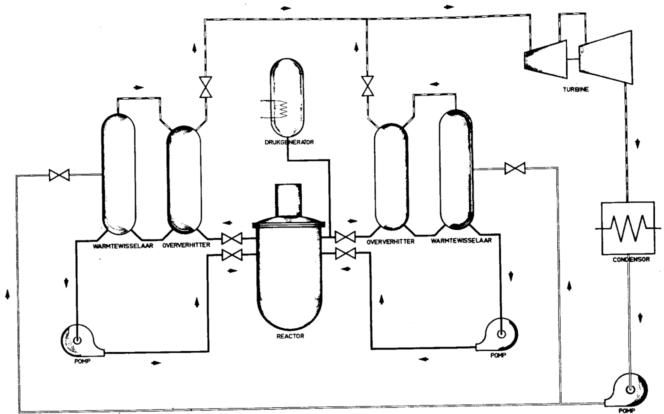
Figuur 1. Principeschema van het primaire systeem dat warmte opneemt in de reactor en weer afstaat in de warmtewisselaars waar stoom gevormd wordt voor de turbine.
