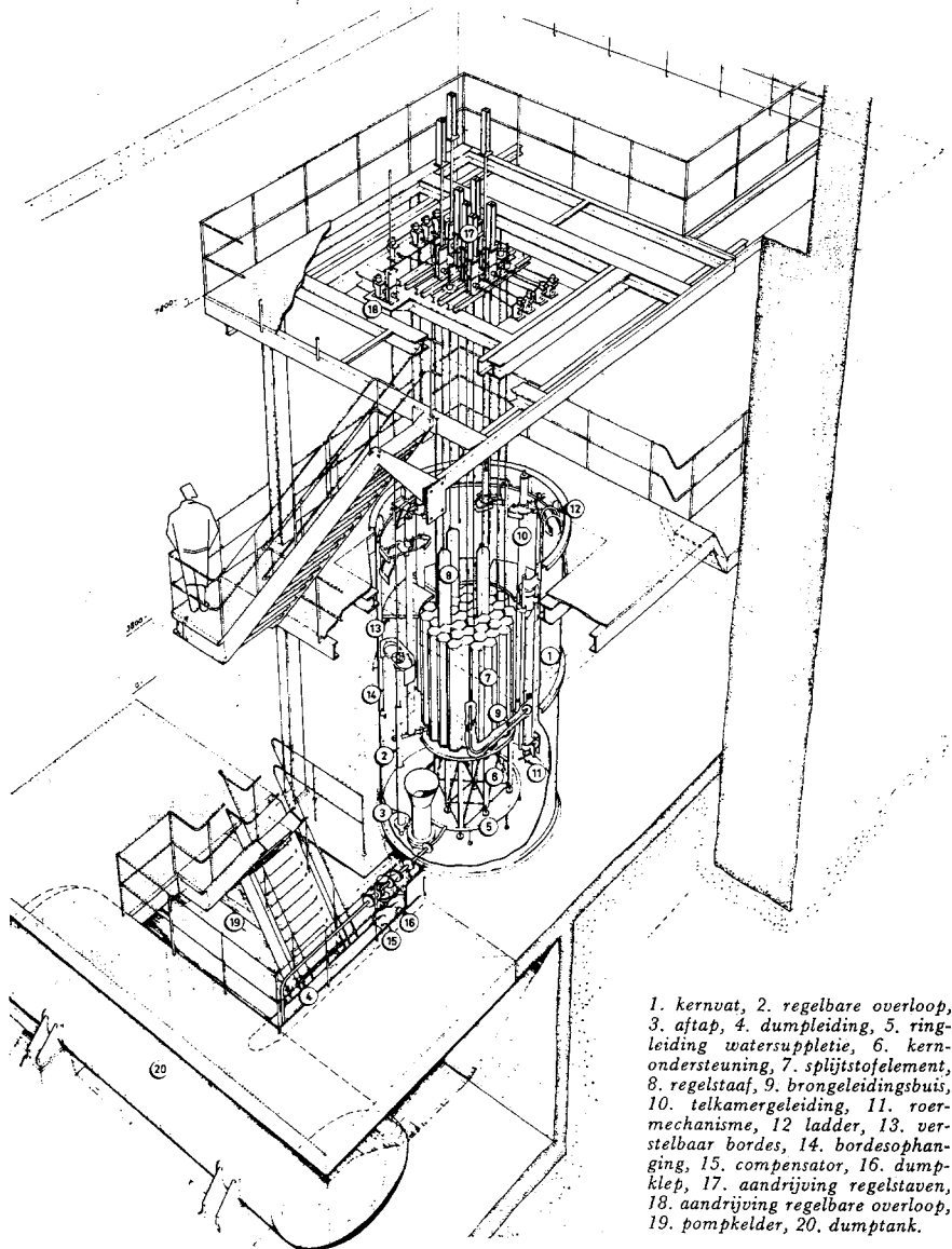
Figuur 3. De installatie waarin kritische experimenten ter bepaling van fysische gegevens over de reactor-kern worden uitgevoerd. Deze installatie ('KRITO') wordt op het terrein van het RCN te Petten opgesteld.
