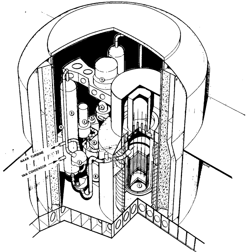
Figuur 2. Het reactorster, 3. warmtewisselaar, 4. circulatiepomp, 5. filters, 6. ionenwisselaars, 7. drukgenerator, 8. afblaastank, 9. spuitank. 1. reactor, 2. oververhitcompartiment vormt een gasdicht omhulsel voor de reactor en de componenten van het primaire systeem.
