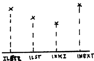
Fig. 7.1: Lokaal minimum
